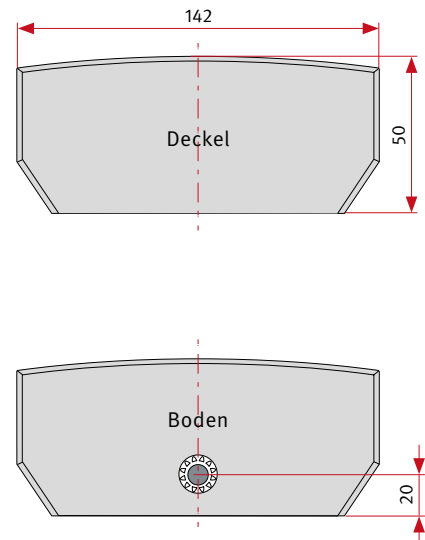
Gehäuse-Deckel und -Boden
