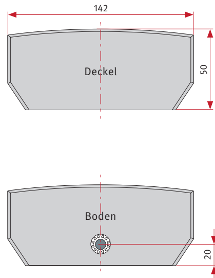
Gehäuse-Deckel und -Boden
