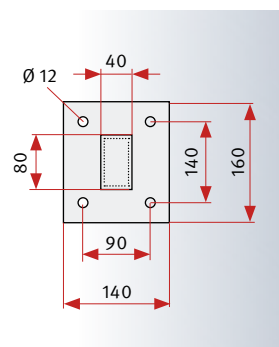
Bodenbefestigung des Pfofens
