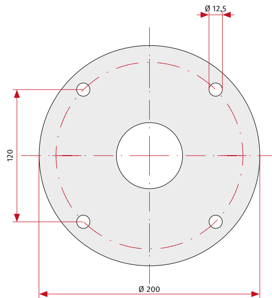
Bodenplatte
